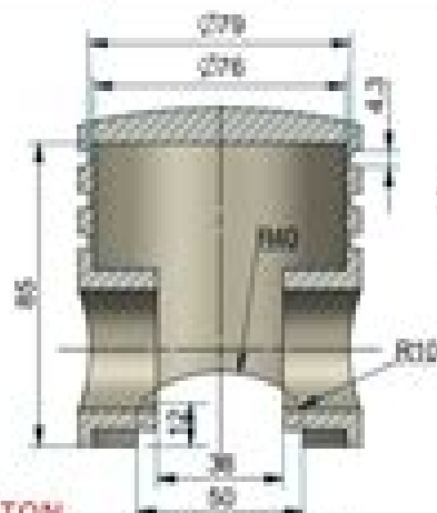
SECTION A-A SCALE 1:1,5
