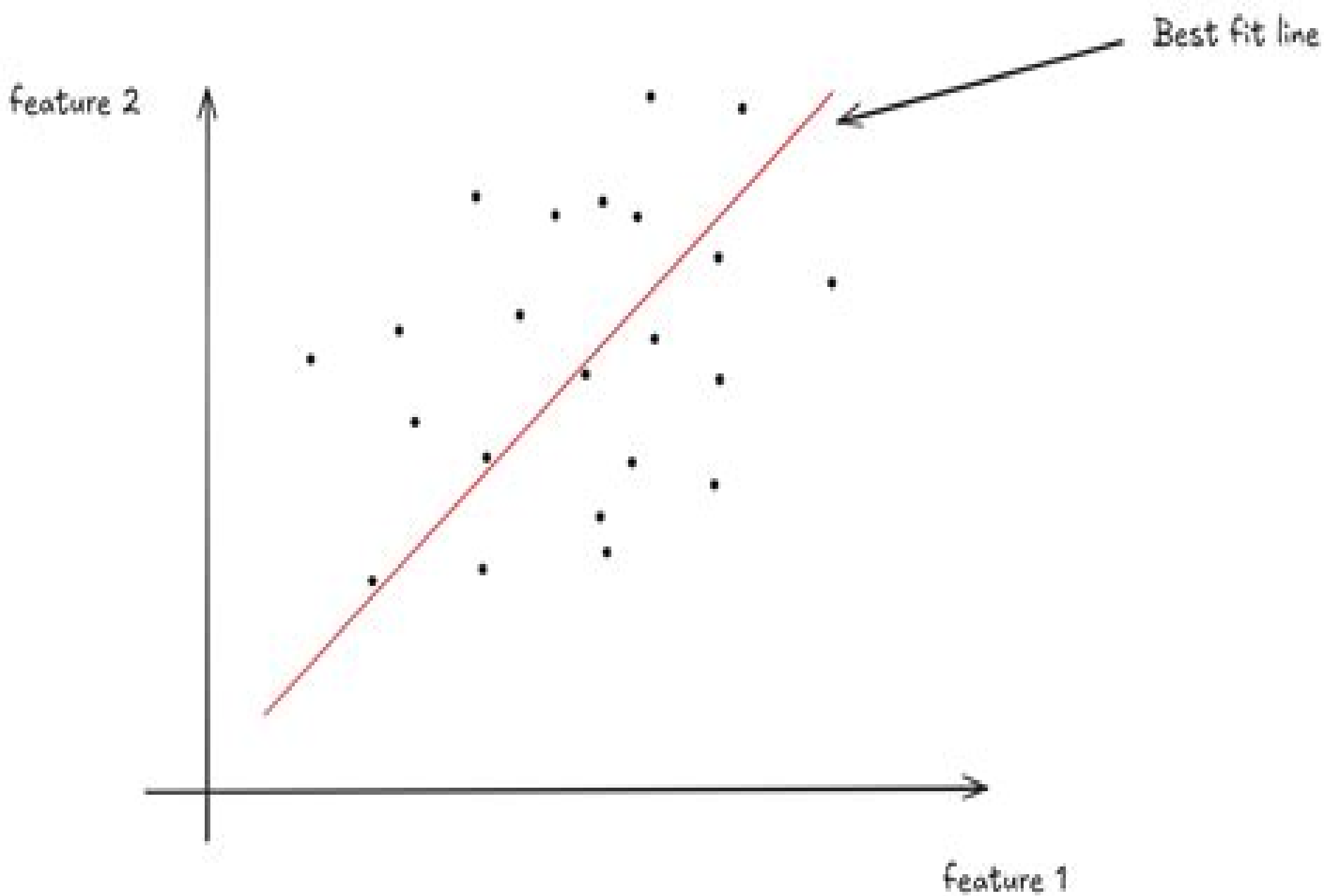
Linear Regression
